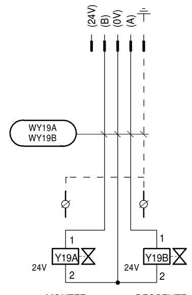
VERIN POINCONNAGE
