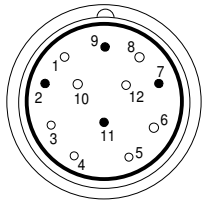
EMBASE MOTEUR
